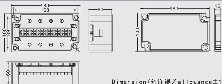
型号 (Model) : DS-PG-15P-M 尺寸 (Size) : 100×180×75mm
