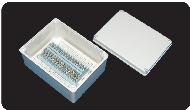
型号 (Model) : DS-AG-30P-S 尺寸 (Size) : 150×200×100mm
