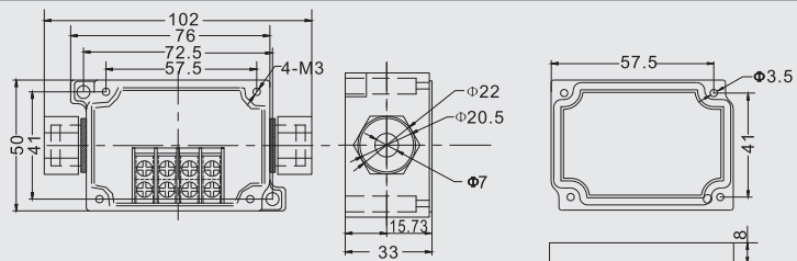
型号 (Model) : DS-MTB-4P 尺寸 (Size) : 50×102×40mm
