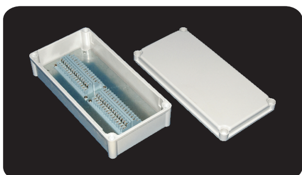
型号 (Model): DS-AG-60P 尺寸 (Size): 380×190×100mm
