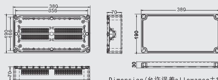
型号 (Model): DS-AG-60P 尺寸 (Size): 380×190×100mm
