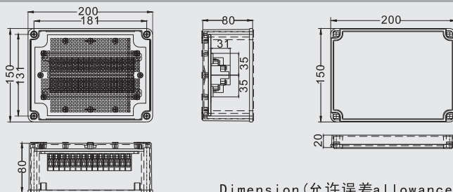
型号 (Model) : DS-AG-30P-S 尺寸 (Size) : 150×200×100mm
