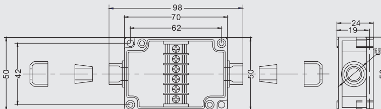
型号 (Model) : PBT-6P 尺寸 (Size) : 50×70×24mm
