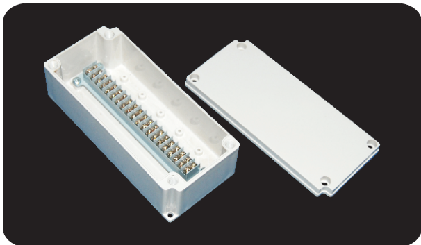
型号 (Model) : DS-PG-20P-M 尺寸 (Size) : 100×223×75
