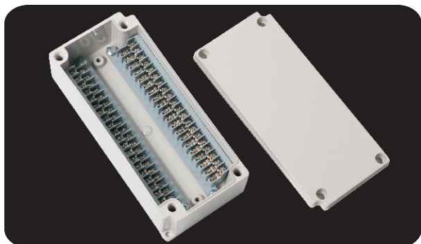
型号 (Model): DS-AG-40P-S1 尺寸 (Size): 100×223×75mm
