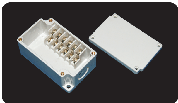
型号 (Model) : DS-6P-K 尺寸 (Size) : 55×91×43mm
