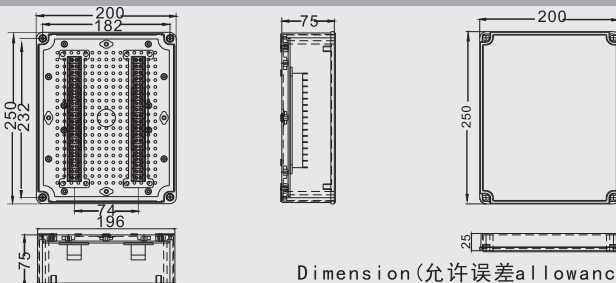
型号 (Model) : DS-AG-40P-M 尺寸 (Size) : 200×250×100mm
