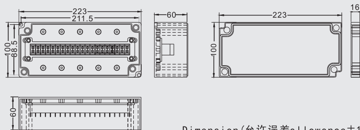
型号 (Model) : DS-PG-20P-M 尺寸 (Size) : 100×223×75
