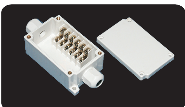
型号 (Model) : DS-MTB-6P 尺寸 (Size) : 55×125×40mm
