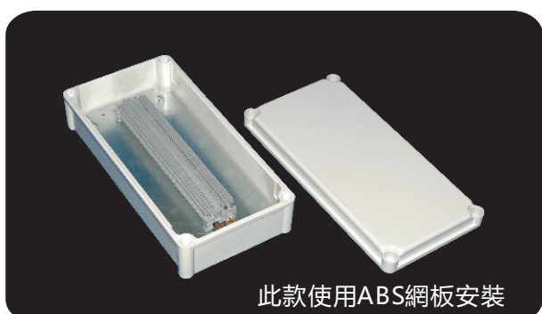
型号 (Model): DS-AG-50P 尺寸 (Size): 380×190×100mm
