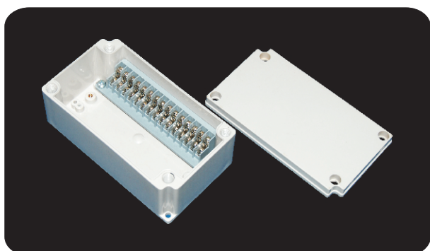
型号 (Model) : DS-PG-15P-S 尺寸 (Size) : 100×180×75mm
