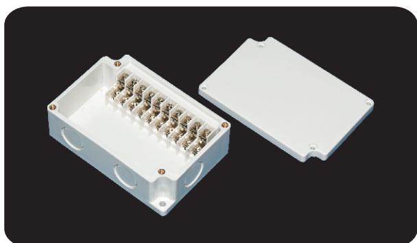
型号 (Model) : DS-PG-10P 尺寸 (Size) : 75×110×40mm
