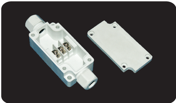
型号 (Model) : PBT-3P 尺寸 (Size) : 33×65×24mm
