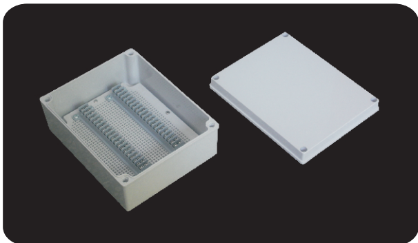
型号 (Model) : DS-AG-40P-M 尺寸 (Size) : 200×250×100mm
