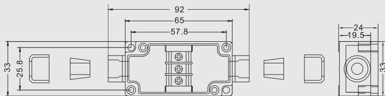
型号 (Model) : PBT-3P 尺寸 (Size) : 33×65×24mm
