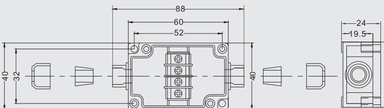
型号 (Model) : PBT-4P 尺寸 (Size) : 40×60×24mm
