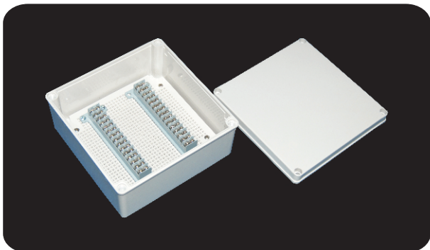
型号 (Model) : DS-AG-30P-M 尺寸 (Size) : 200×200×95mm
