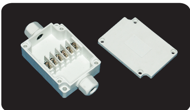
型号 (Model) : PBT-6P 尺寸 (Size) : 50×70×24mm
