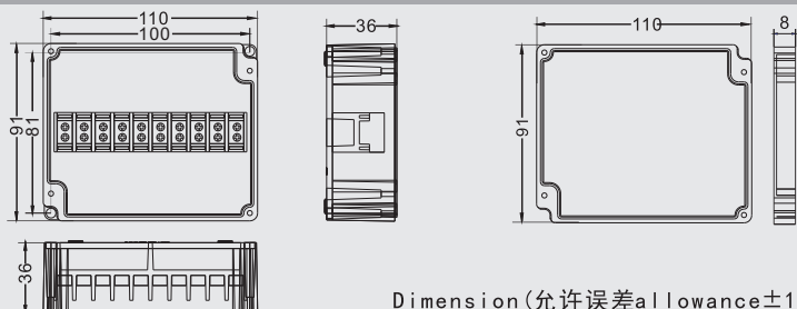
型号 (Model) : DS-10P-M 尺寸 (Size) : 91×110×43mm
