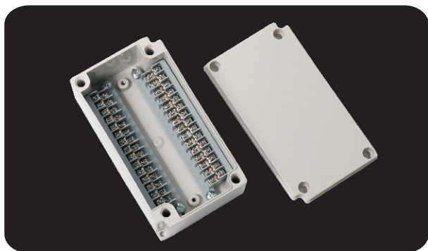
型号 (Model): DS-AG-30P-S1 尺寸 (Size): 100×180×75mm
