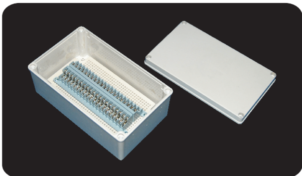
型号 (Model) : DS-AG-40P-S 尺寸 (Size) : 150×250×100mm
