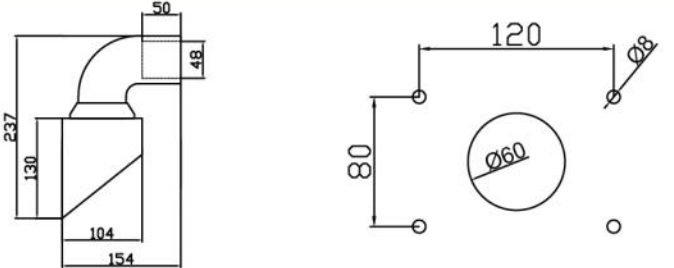
品名：水平牆座 訂貨號：4860 重量：3.2kg 材料：不鏽鋼可旋轉320°
