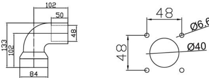
品名：90°箱體連接器 訂貨號：4850 重量：2.3kg 材料：不鏽鋼可旋轉320°
