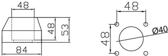
品名：內裝固定底座 訂貨號：4840 重量：1.1kg 材料：不鏽鋼可旋轉320°
